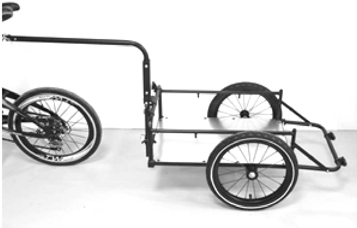
B71-061V02/B71-061V03 (com placa inferior galvanizada)
