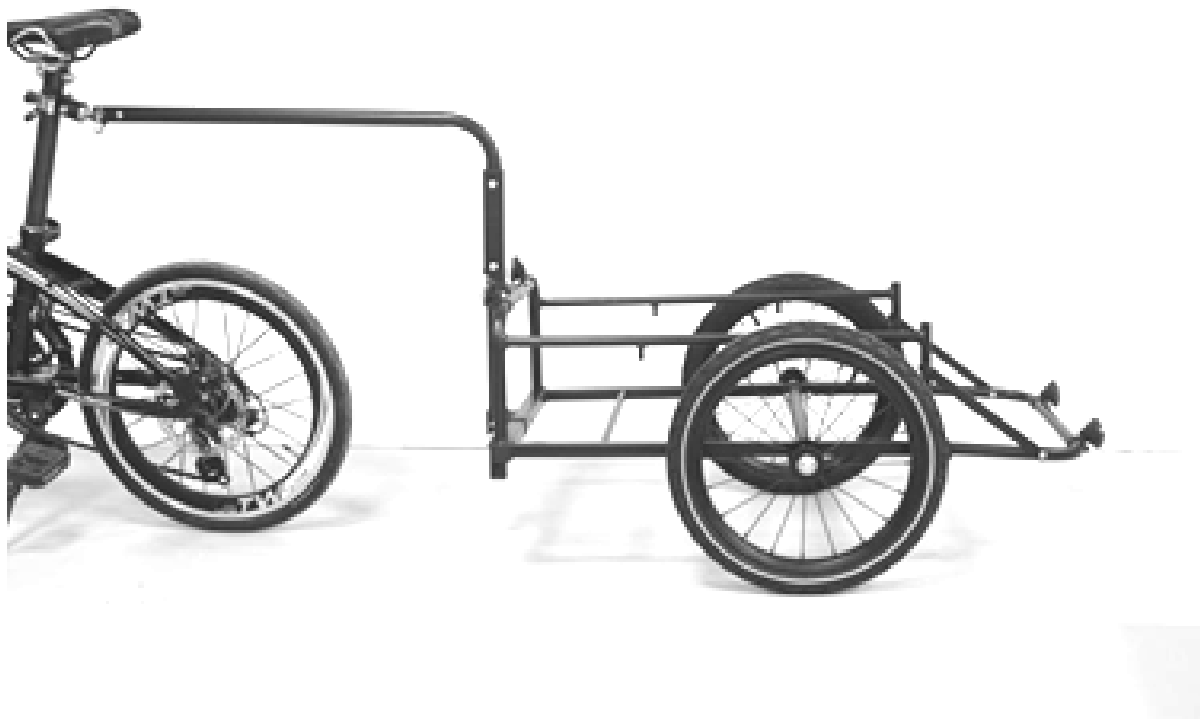
B71-061V00/B71-061V01 (ohne verzinkte Bodenplatte)
