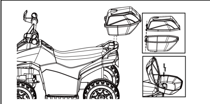
7.Fix the trunk (3X(4X10)SCREW)
